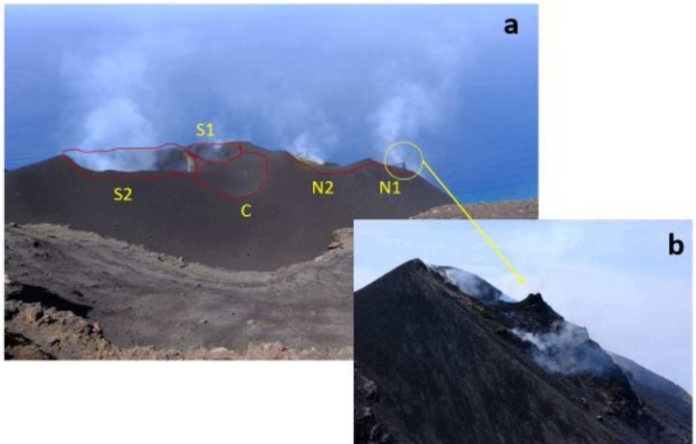
Fig. 3.3 a) Panoramica della terrazza craterica vista dal Pizzo con la delimitazione e la denominazione dei settori, b) Hornito del settore N1
