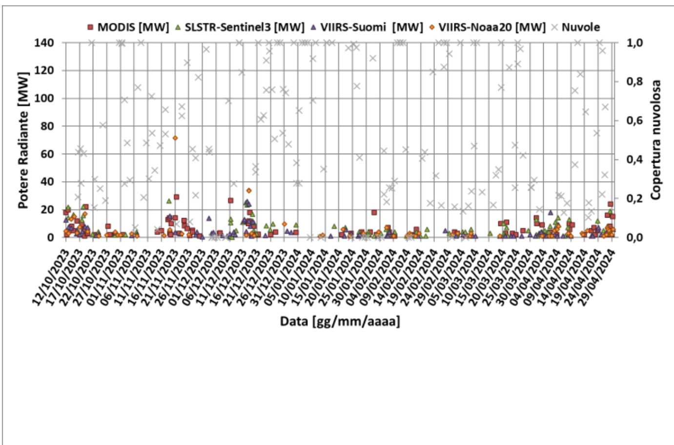
Fig. 7.1 Potere radiante calcolato da dati MODIS (quadrato rosso), SENTINEL-3 SLSTR (triangolo verde) e VIIRS (triangolo viola e rombo giallo) dal 12 ottobre 2023 al 29 aprile 2024. Per l'intero periodo analizzato è anche riportato l'indice di nuvolosità.
